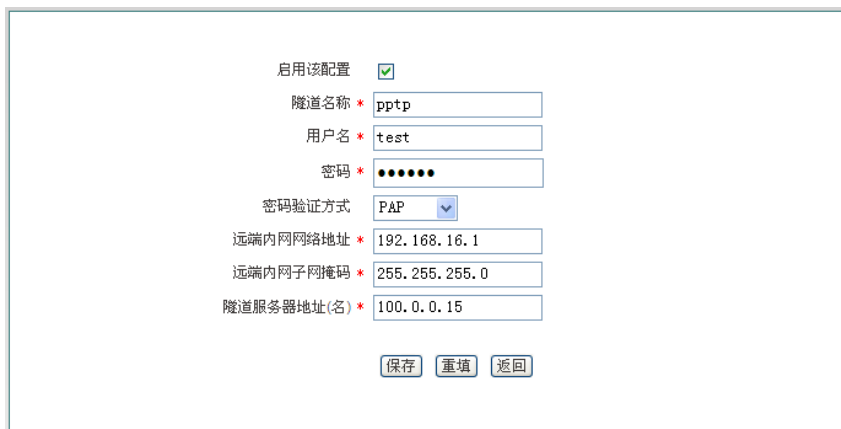
图 12-5 PPTP 客户端
