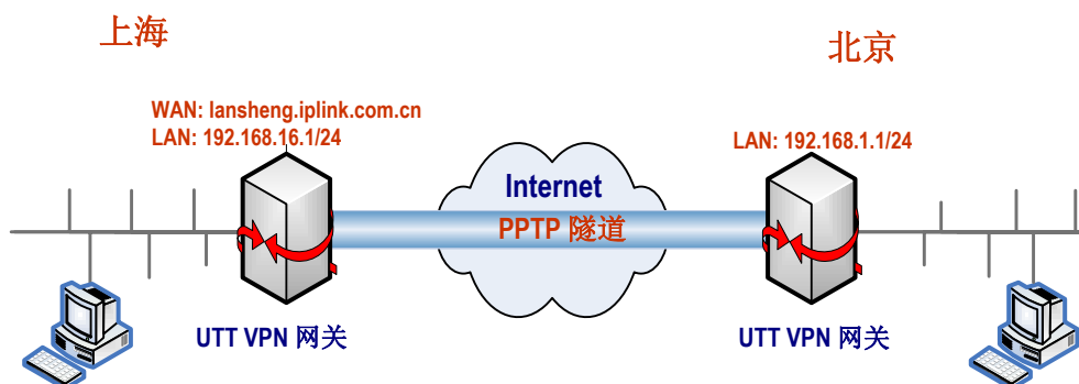
图 12-6 PPTP 实例拓扑图
